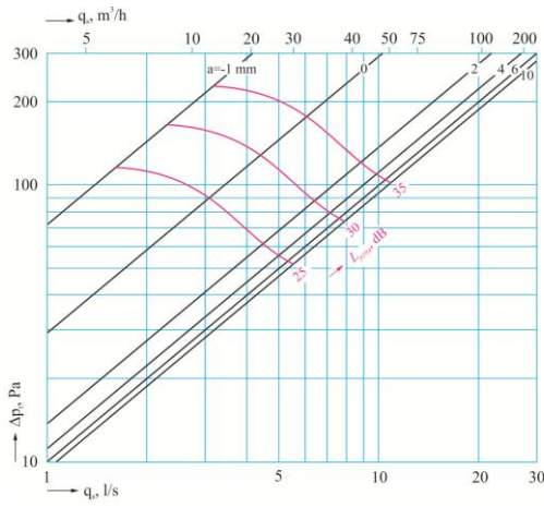
DVS-PY 080 mm
